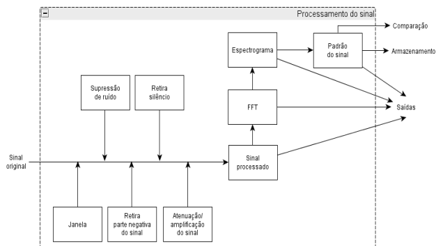
Figura 4: Diagrama de blocos da etapa de processamento do sinal.
