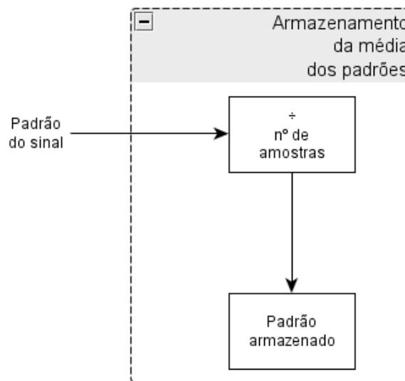
Figura 6: Diagrama de blocos representando a forma de armazenamento dos padrões amostrados.
